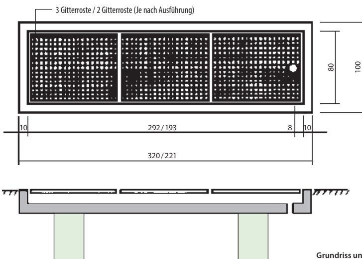
Grundriss und Schnitt
